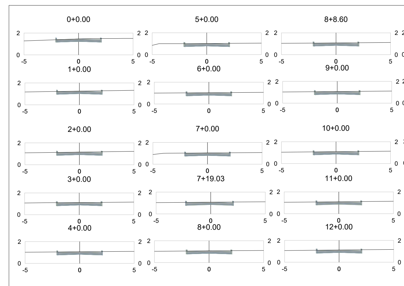
Perfil Transversal - Rua Santo Antônio Escala ——— 1:1000
