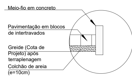
Detalhe 01 Escala ——— 1:25
