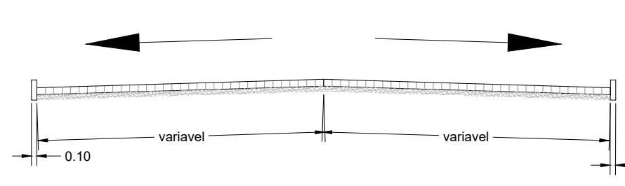
Seção Transversal Tipo Escala ——— 1:100
